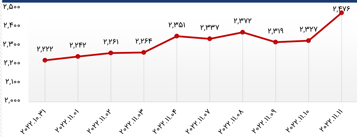
نمودار (۱۹): قیمت جهانی یک تن آلومینیوم در روزهای هفته منتهی به ۱۴۰۱/۰۸/۲۰ و هفته قبل از آن (دلار)
